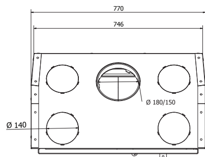
Bovenaanzicht / Vue de dessus
