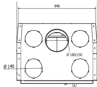
Bovenaanzicht / Vue de dessus
